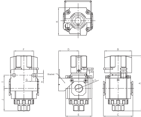
진압배기밸브
