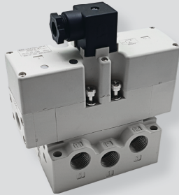
EN175301-803:2006 (구 DIN 43650 A) 콘넥터 V/V
