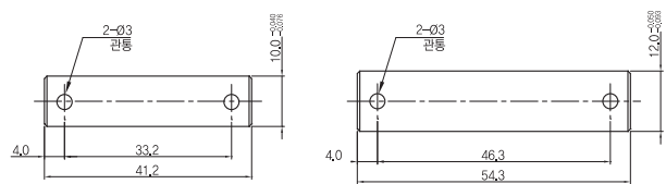
클래비스용 핀,너클용 핀 (Ø40)
