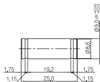
클래비스용 핀, 너클용 핀(Ø20,25,32)
